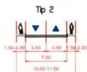
PRESJEK D__D
