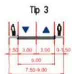
PRESJEK C__C
